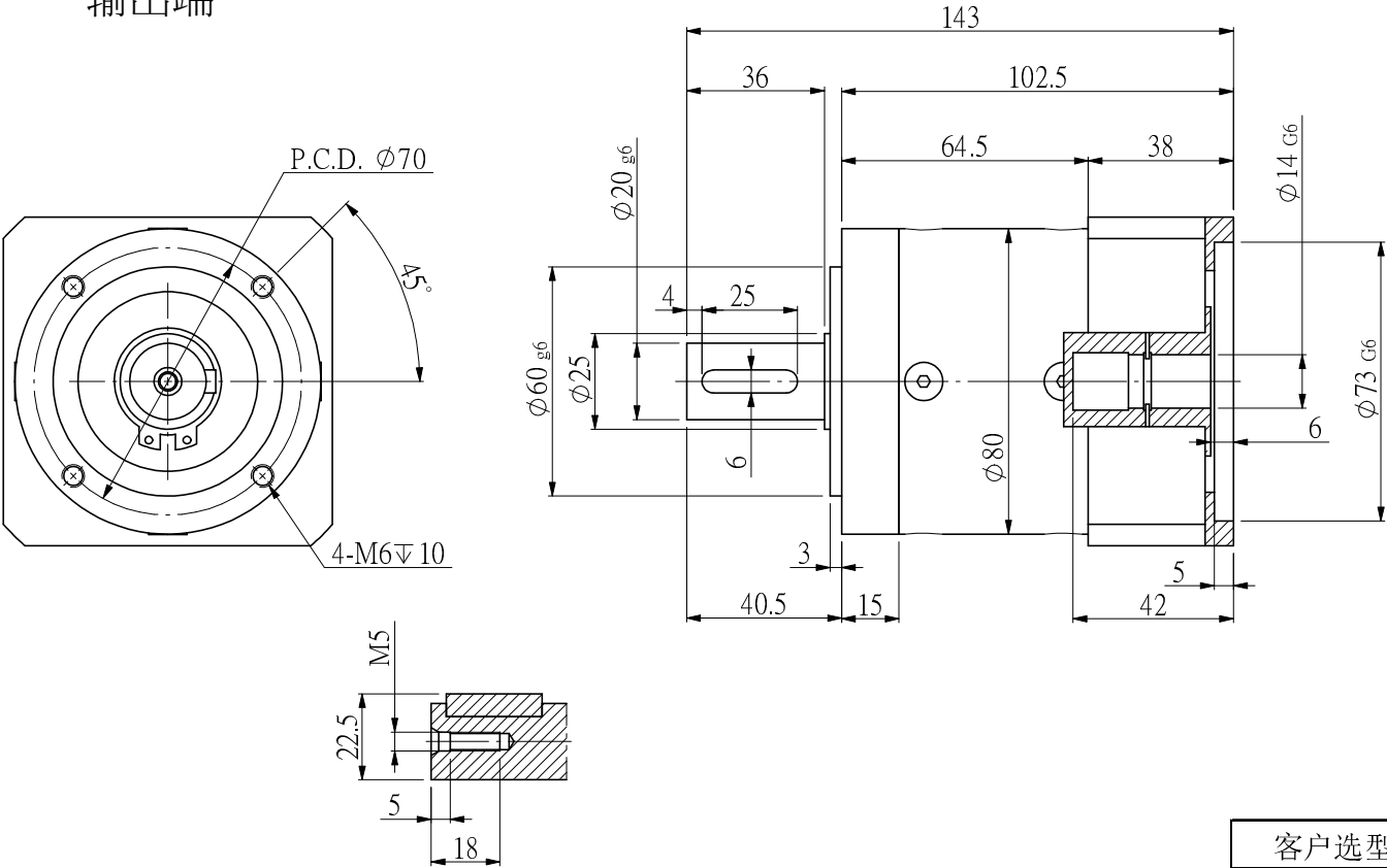
输出端
