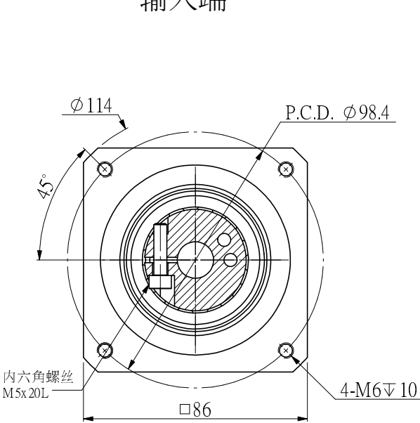
输入端
